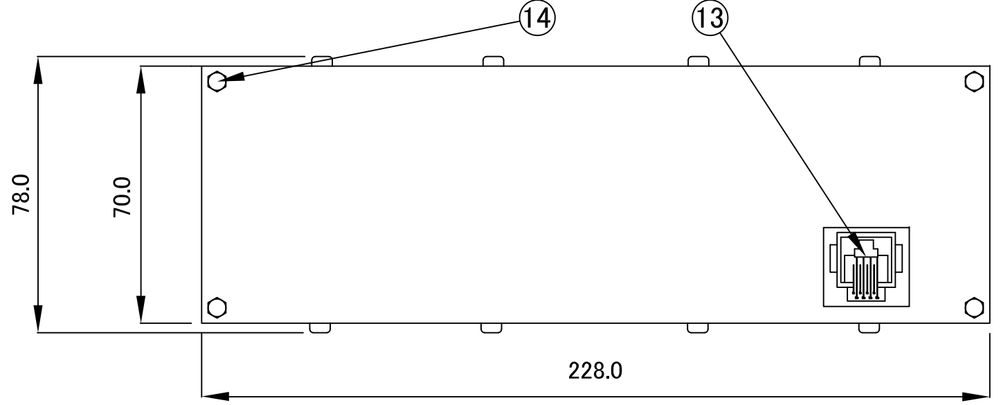
開口寸法・取付け穴
